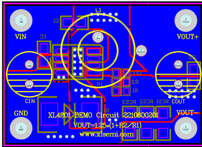
底层
